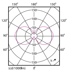
(cd/1000lm) 0^\circ
