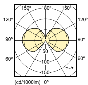
(cd/1000lm) 0°
