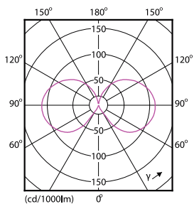
(cd/1000lm) 0°
