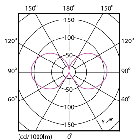
(cd/1000lm) 0°
