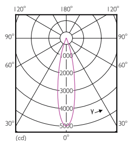
PAR30L 12W 850lm 40D 2700K E26
