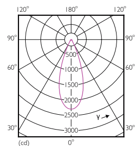
PAR30L 12W 950lm 40D 4000K E26
