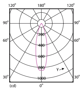
LEDspot PAR20 7W 822 827 500lm 25D
