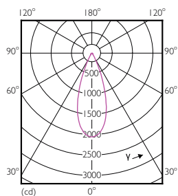
PAR30L 12W 950lm 25D 4000K E26
