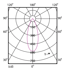
LEDspot PAR20 7W 830 500lm 40D
