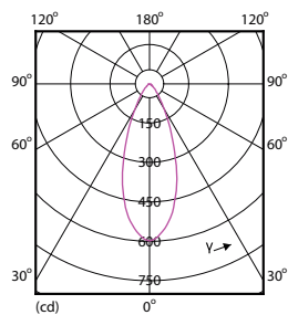
LEDspot PAR20 7W 840 500lm 40D
