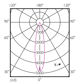
PAR30L 12W 850lm 25D 2700K E26
