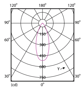
LEDspot PAR20 7W 822 827 500lm 40D
