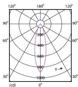
LEDspot PAR20 7W 840 500lm 25D
