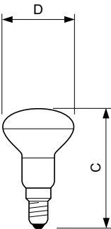
REF STD 30W E14 240-250V R39 45D FR
