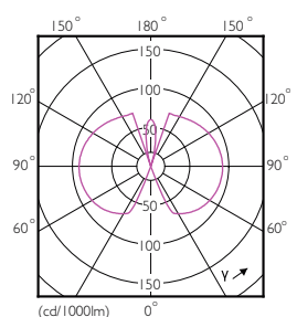
Bulb G25 120V 350lm 150D 5000K E26 ND
