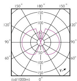
Bulb G25 120V 350lm 150D WW E26 ND
