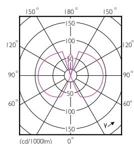
Bulb G25 120V 500lm 150D 5000K E26 ND
