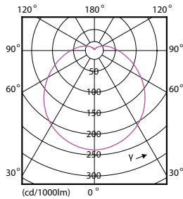
LEDbulb 150W E27 827 FR A80
